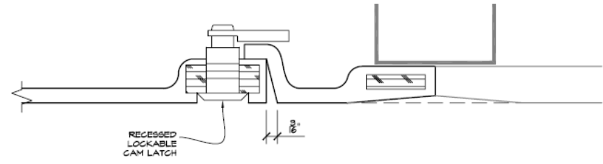
SECTION VIEW Scale: 6"=1'
