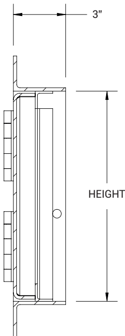
SECTION A-A
